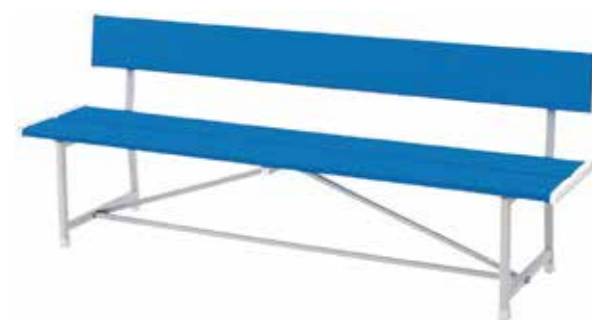
Y-T1373 コートベンチ180スチール(青・緑) 本体価格(1台) ¥97,900(税込) 寸法/長さ1805×巾450×高さ390mm 仕様/組立式・フレーム スチール・座面 再生ABS成形品 重量/22kg 運/見積
